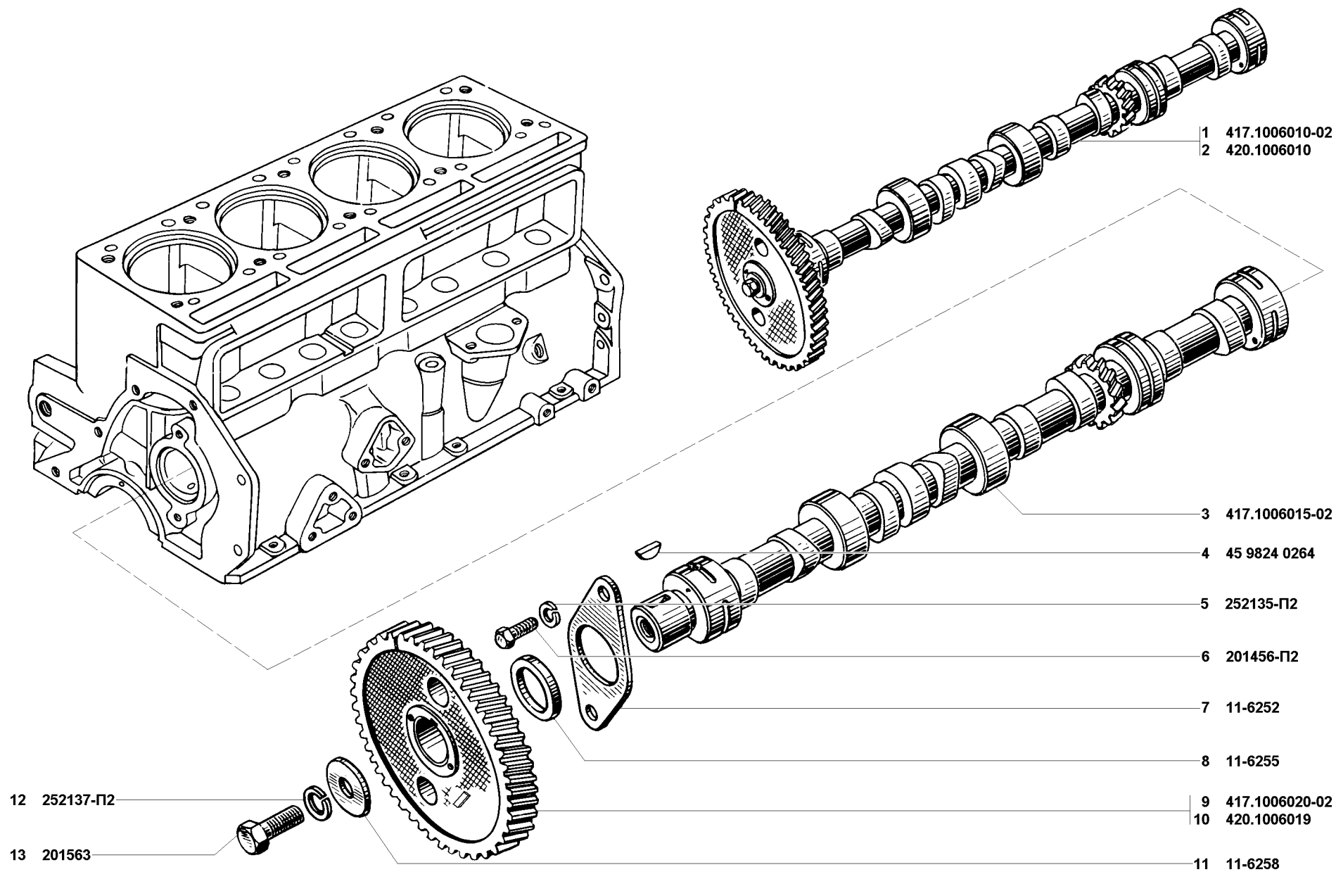
Рис. 7. Вал распределительный (1006)
